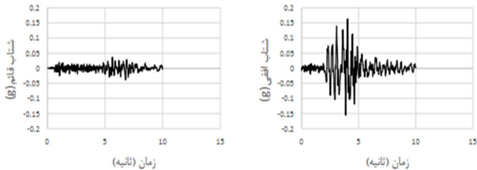
شکل (۹): شتاب نگاشت مؤلفه افقی و قائم زلزله نورترین کالیف
