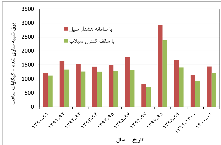
شکل (۶): تولید برق شبیه سازی شده با سامانه هشدار سیل و سقف کنترل سیلاب در نیروگاه برق آبی سد کارون ۴
