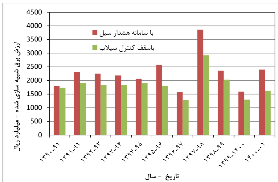
شکل (۷): ارزش برق با سامانه هشدار سیل و سقف کنترل سیلاب در نیروگاه برق آبی سد کارون ۴
