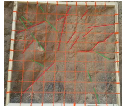
شکل (۶): اندازه‌گیری چگالی درزه‌داری سطحی ( P_{20} ) با
