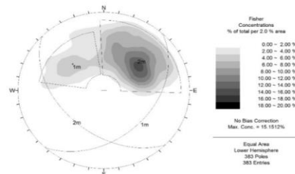
شکل (۷): تفکیک دسته‌درزه‌های برداشت‌شده از بخش‌های
