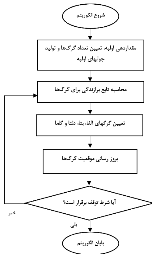
شکل (۲): فلوجارت کلی الگوریتم گرگ خاکستری
