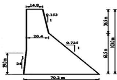
شکل (۱): ابعاد هندسی مقطع عرضی سد بتنی وزنی کوینا
