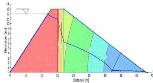
شکل (۷): تعیین خط فریاتیگ با کاهش نفوذپذیری
