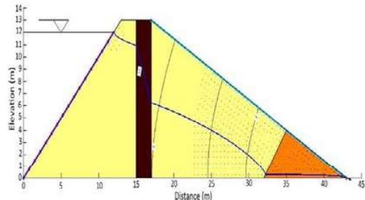
شکل (۸): تعیین خط فریاتیگ با افزایش نفوذپذیری
