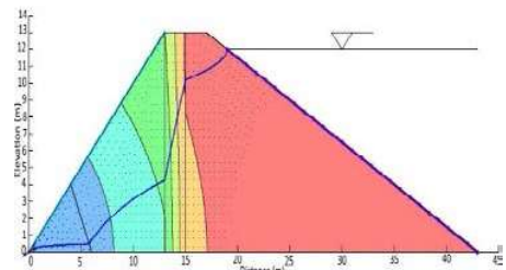
شکل (۱۴): نمایش خط فریاتیگ در حالت جابجایی بالادست و پایین دست
