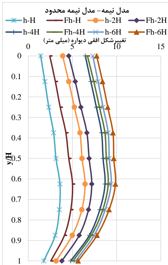
شکل (۱۹): مقایسه تغییر شکل افقی در مقطع بحرانی دیوار میخکوبی شده ۸ متری الف- مدل کامل و مدل نیمه (ب) - مدل نیمه و مدل نیمه محدود
