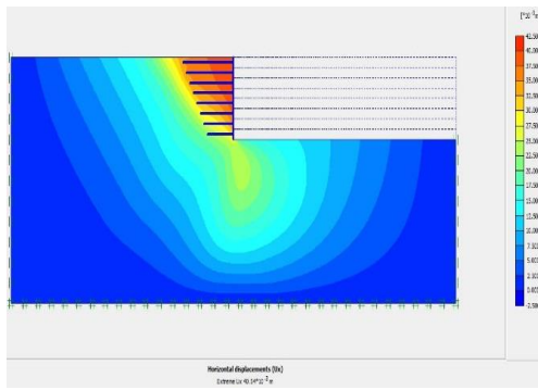
شکل (۸): کانتور تغییر شکل افقی دیوار میخکوبی شده به ارتفاع ۱۶ متر در آخرین مرحله خاک برداری
