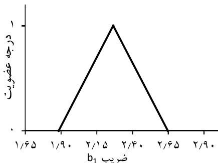
شکل (۸): توابع عضویت مثلثی ضرایب رابطه منحنی سنجھ بار معلق، b_1
