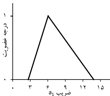
شکل (۷): تابع عضویت مثلثی ضرایب رابطه منحنی سنجھ بار معلق، a_1
