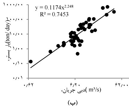
شکل (۶): منحنی سنجھ رسوب سالانه، (الف): بار معلق، (ب): بار بستر، (log-log)
