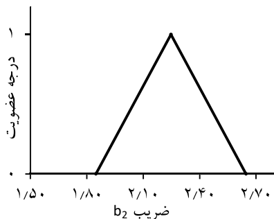
شکل (۱۰): تابع عضویت ضرایب رابطه منحنی سنجھ بار بستر، (الف) a_2 و (ب) b_2
