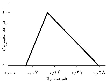
شکل (۹): تابع عضویت ضریب رابطه منحنی سنجھ بار بستر، a_2
