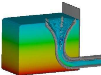
ج) سرریز با شش تیهه گرداب شکن
