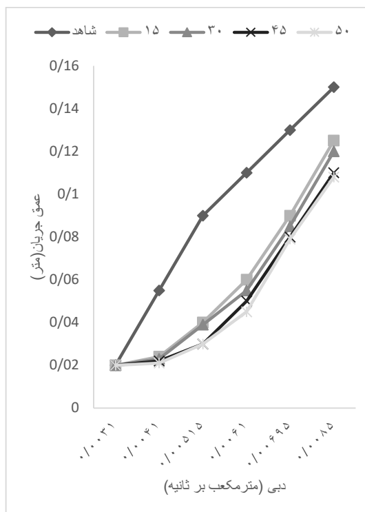
شکل (۲۱): نمودار دبی- اشل برای آرایش ۶ تیغه گردابه‌شکن
