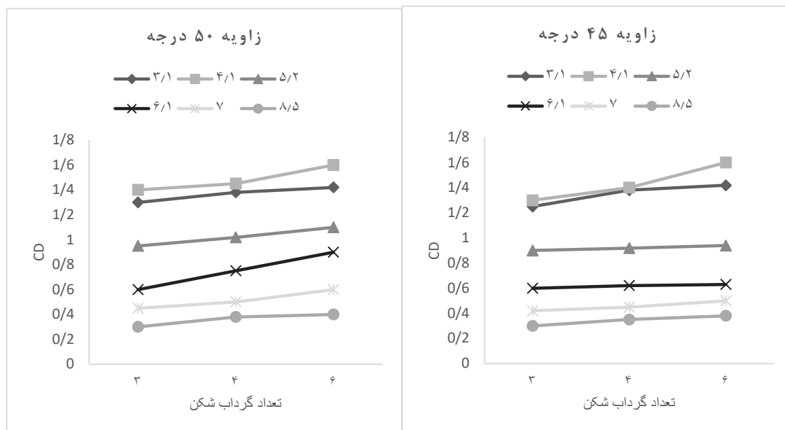
شکل (۲۷): نمودار ضریب دبی - تعداد گرداب شکن‌ها با زاویه ی ۵۰-۴۵-۳۰-۱۵ درجه
