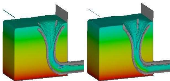
الف) سرریز با سه تیهه گرداب شکن ب) سرریز با چهار تیهه گرداب شکن
