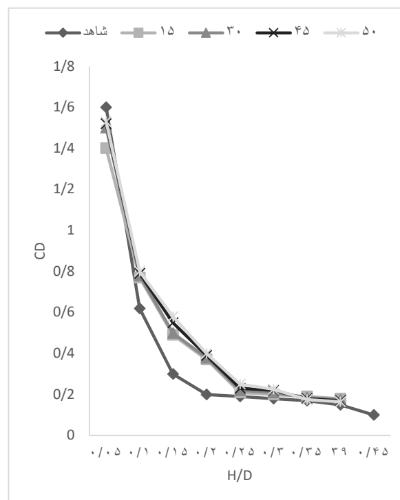
شکل (۲۵): نمودار ضریب دبی - نسبت
