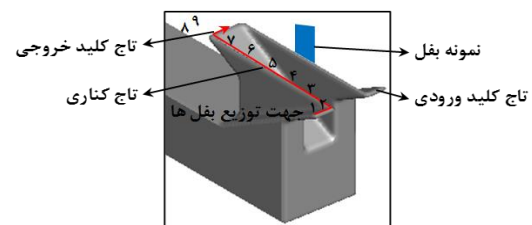
شکل (۱۳): موقعیت قرارگیری بفل‌ها در مدل عددی
