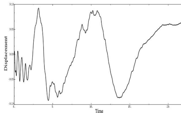
شکل (۷): نمودار جابجایی (متر) نقطه روی سمت راست (نقطه C) تحت جنبش یکنواخت.
