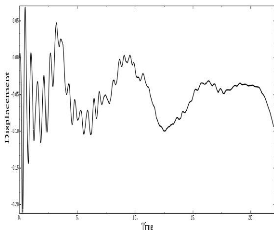
شکل (۵): نمودار جابجایی (متر) تاج سد (نقطه A) تحت جنبش یکنواخت (متر).
