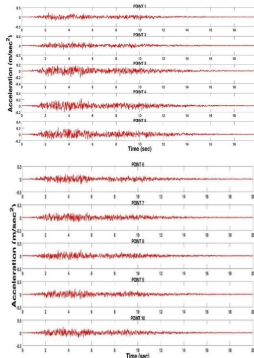
شکل (۱): شتاب‌های تولیدشده بر روی سنگ بستر
