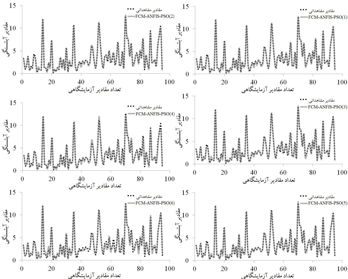
شکل (۷): مقایسه مقادیر آبخستگی مشاهداتی (ds/dw) و شبیه‌سازی شده برای مدل‌های مختلف FCM-ANFIS-PSO
