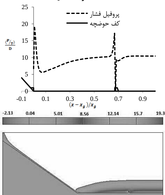
شکل (۶): پروفیل بی‌بعد فشار در کف حوضچه نوع II
