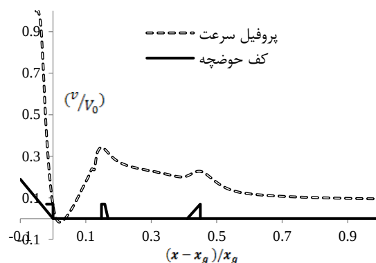
شکل (۱۱): پروفیل بی‌بعد سرعت در حوضچه نوع III ( x_g=2/39 ) ( Q=0/113 و v_0=5/34 )
