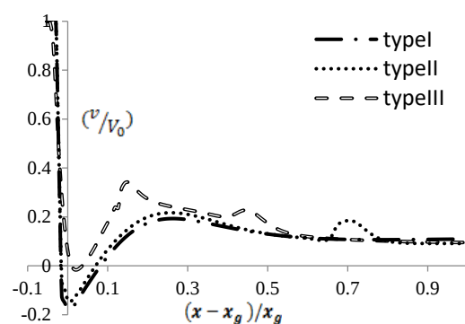
شکل (۱۲): پروفیل بی‌بعد سرعت سه حوضچه ( x_g=2/39 ) و ( Q=0/113 )
