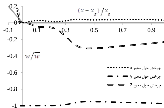
شکل (۱۴): پروفیل بی‌بعد چرخش در حوضچه نوع I X_g=2/39 و (Q=0/113)
