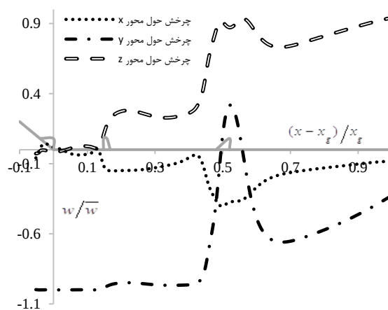
شکل (۱۶): پروفیل بی‌بعد چرخش در حوضچه نوع III X_g=2/39 و (Q=0/113)
