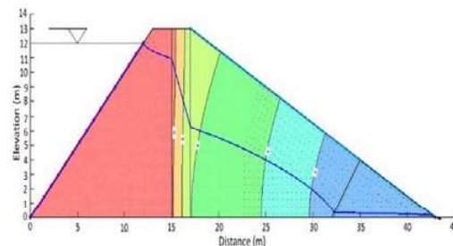
شکل (۷): تعیین خط فریاتیک با کاهش نفوذپذیری‌ها
