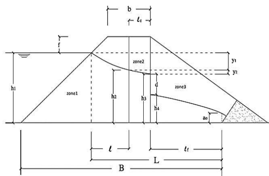
شکل (۱): مدل هندسی مطالعاتی رزک برای سد خاکی با هسته داخلی
