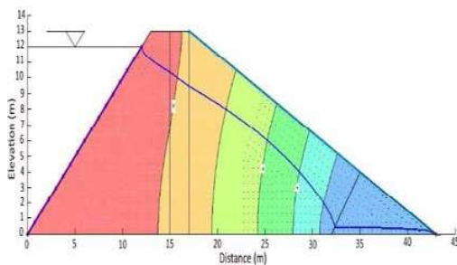
شکل (۱۰): خط فریاتیک در نسبت k_c/k_d = 0.8
