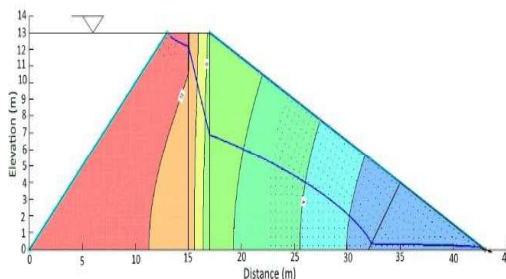
شکل (۱۲): نمایش خط فریاتیک با افزایش ارتفاع سطح آب
