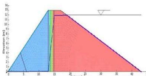
شکل (۱۶): نمایش خط فریاتیگ با نسبت K_c/K_d = 0.001
