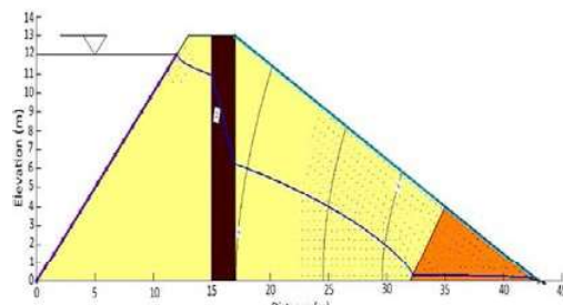
شکل (۸): تعیین خط فریاتیک با افزایش نفوذپذیری‌ها
