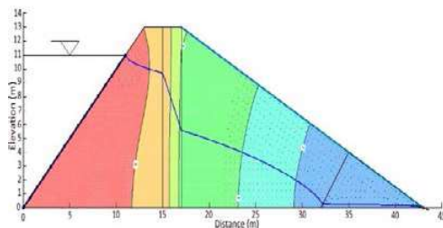
شکل (۱۱): نمایش خط فریاتیک با کاهش ارتفاع سطح آب
