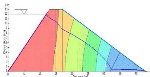
شکل (۱۲): نمایش خط فریاتیک با افزایش ارتفاع سطح آب
