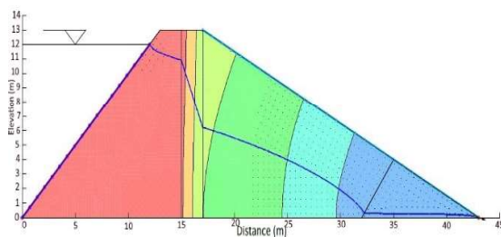
شکل (۵): نحوه توزیع فشار آب منفذی و خط فریاتیک در سد
