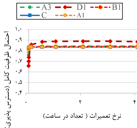
شکل (۱۴): حساسیت احتمال ظرفیت کامل نیروگاه به نرخ تعمیرات تجهیزات
