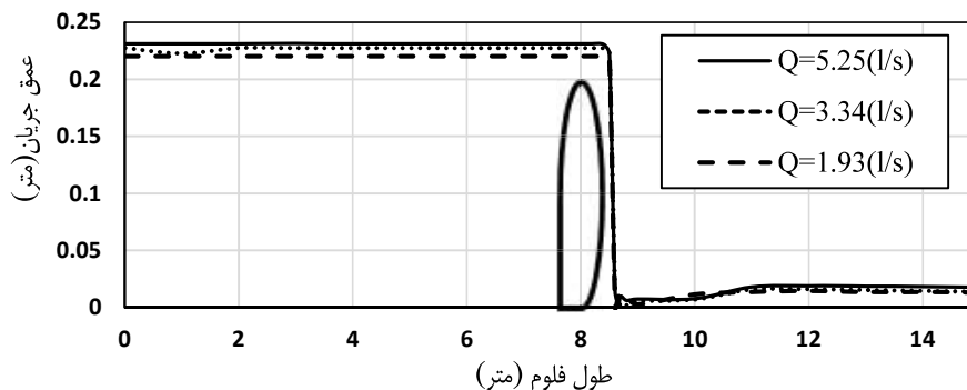
شکل (۱۱): رابطه میزان فشار درون تیوپ سد لاستیکی بر عمق جریان ( p=3 KN/m²)
