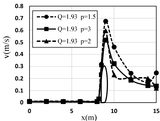
شکل (۱۳): نمایش سرعت متوسط جریان در (Q=1.93 \text{ l/s})
