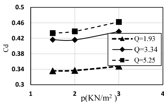
شکل (۹): رابطه ضریب دبی با فشار درون تیوپ سد
