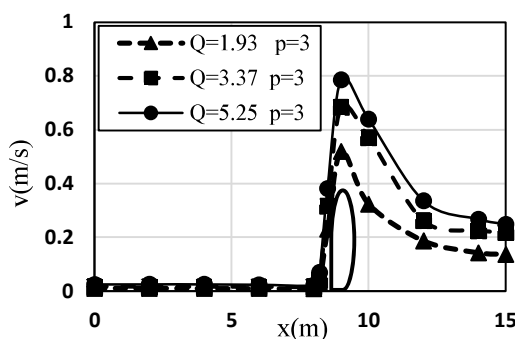
شکل (۱۶): نمایش سرعت متوسط جریان در P=3 \text{ KN/m}^2
