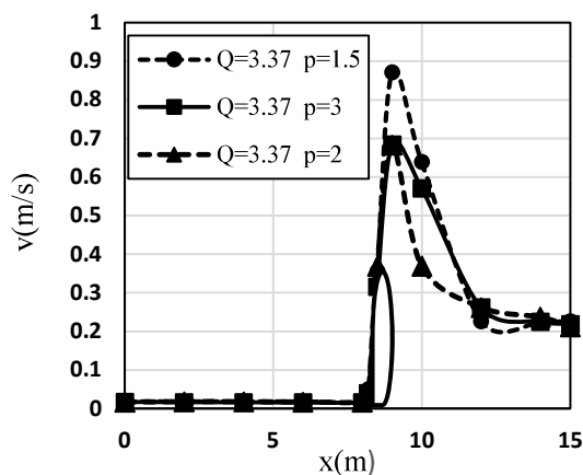
شکل (۱۴): نمایش سرعت متوسط جریان در (Q=3.37 \text{ l/s})
