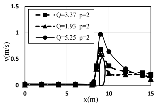
شکل (۱۵): نمایش سرعت متوسط جریان در P=2 \text{ KN/m}^2
