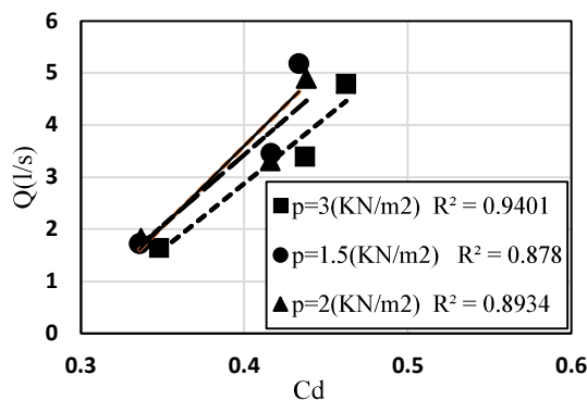
شکل (۶): رابطه دبی با ضریب دبی
