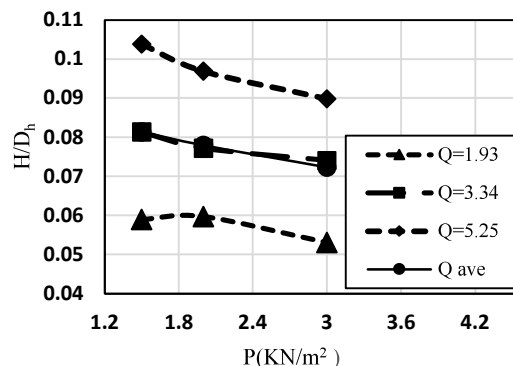
شکل (۸): رابطه فشار درون تیوپ با H/D_h
