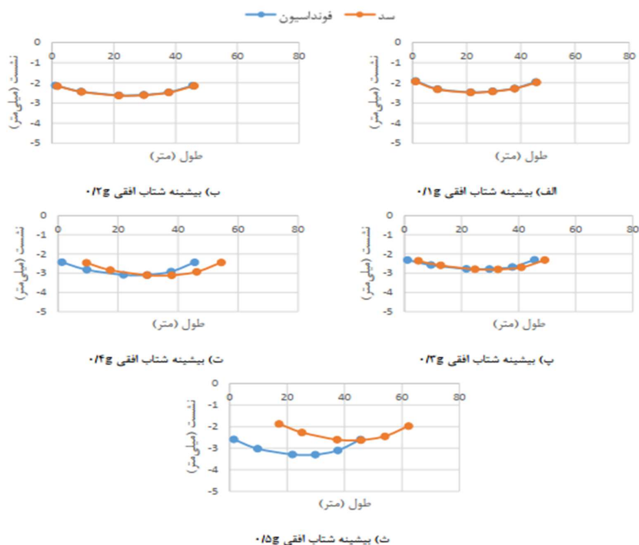
شکل (۱۳): تغییر شکل سطح تماس سد و فونداسیون تحت زلزله آنرا
