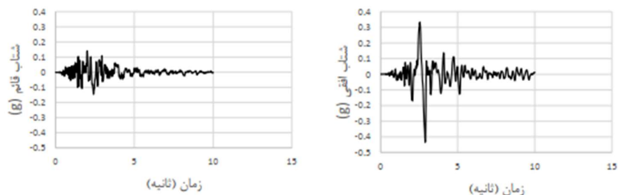
شکل (۷): شتاب‌نگاشت مؤلفه افقی و قائم زلزله کوپوت لیک
