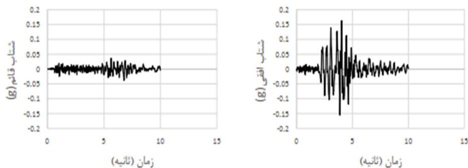
شکل (۹): شتاب نگاشت مؤلفه افقی و قائم زلزله نورترن کالیف
