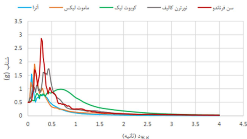
شکل (۱۰): طیف شتاب زلزله‌ها
