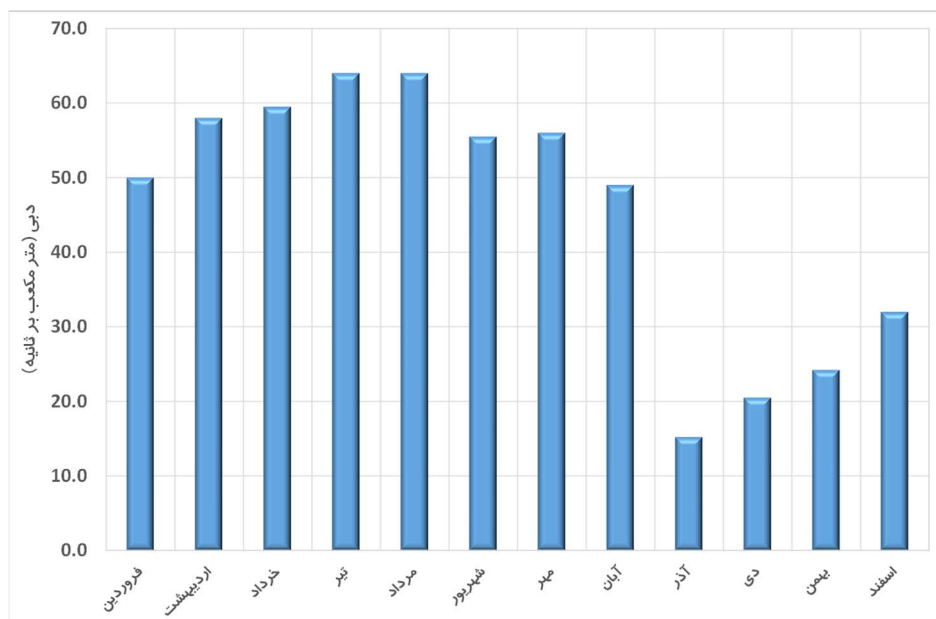
شکل (۲): توزیع ماهانه مجموع برداشت آبگیرهای چپ و راست سد تنظیمی گتوند
