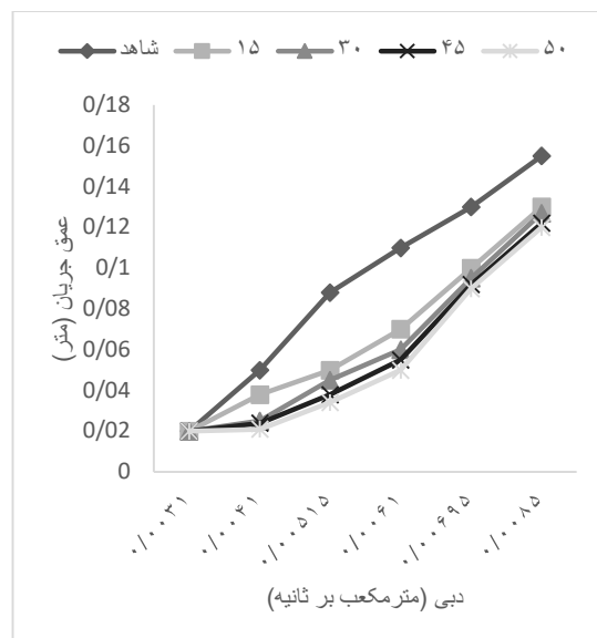
شکل (۲۰): نمودار دبی - اشل برای آرایش ۴ تیغه
