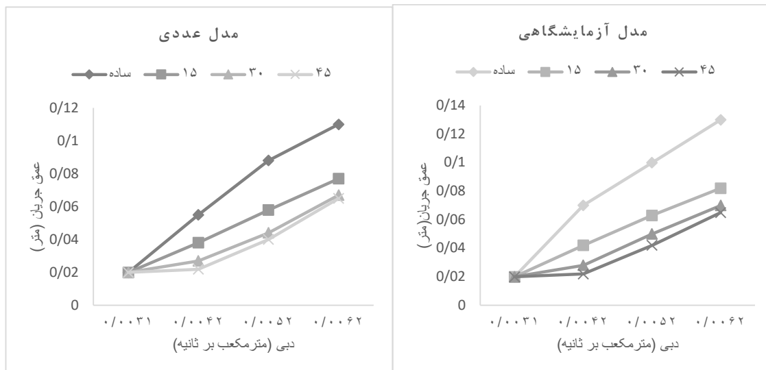
شکل (۱۱): نمودار دبی- اشل سرریز با ۳ تیغه گردابشکن در مدل و آزمایشگاهی
