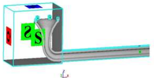
شکل (۸): سرریز نیلوفری با تیغه‌های گرداب شکن در فضای
