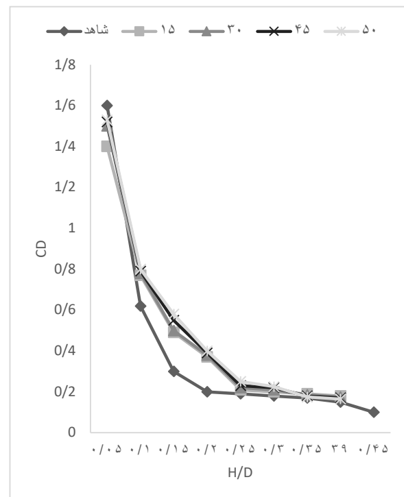
شکل (۲۵): نمودار ضریب دبی - نسبت
