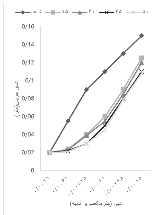
شکل (۲۱): نمودار دبی- اشل برای آرایش ۶ تیغه گردابه‌شکن
