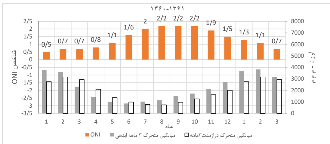
شکل (۷): میانگین متحرک ۳ ماهه و درازمدت ۳ ماهه‌ی آورد حوضه‌ی کارون و شاخص ONI در ال نینو سال ۱۳۶۰-۶۱
