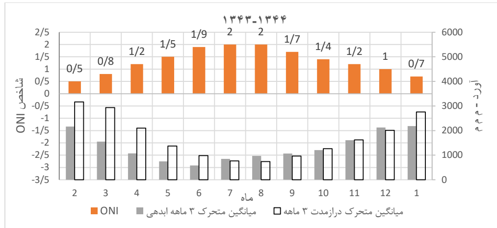
شکل (۵): میانگین متحرک ۳ ماهه و درازمدت ۳ ماهه‌ی آورد حوضه‌ی کارون و شاخص ONI در ال نینو سال ۱۳۴۳-۴۴
