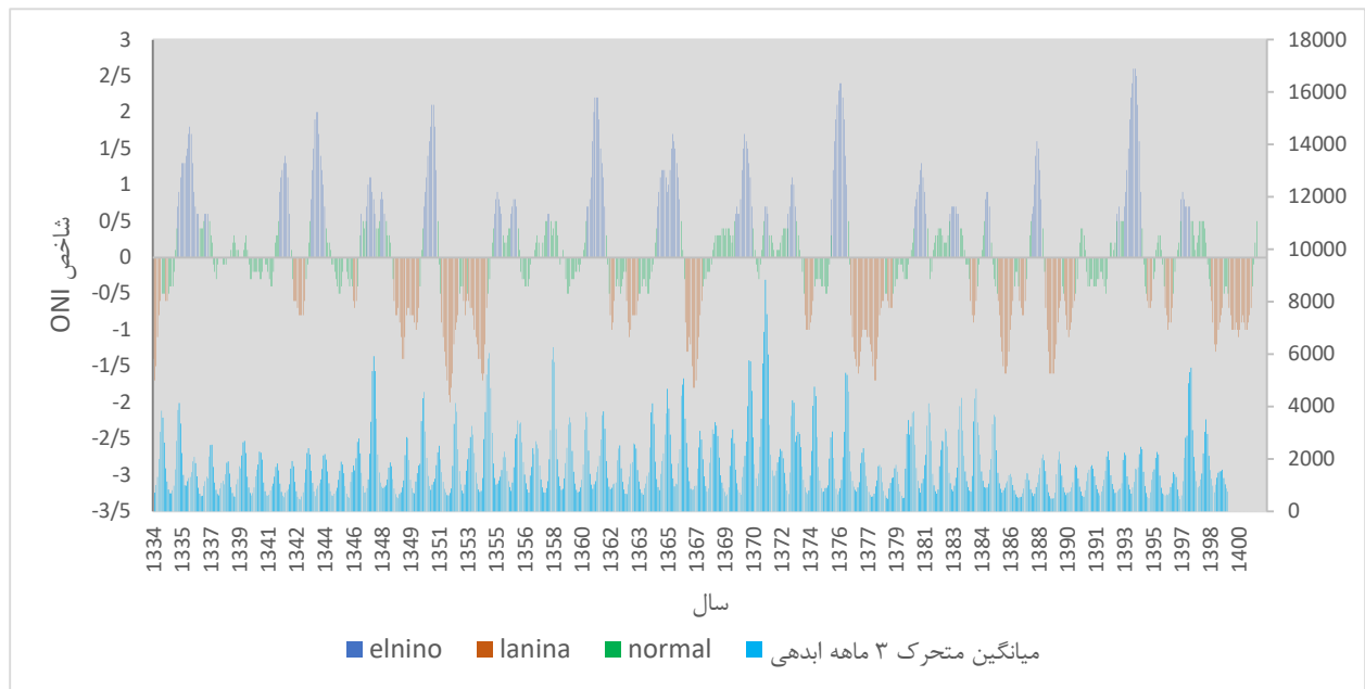
شکل ۳: دوره‌های ال‌نینو و لانینا به همراه میانگین متحرک ۳ ماهه ابدی حوضه‌ی کارون در دوره‌ی آماری مشترک
