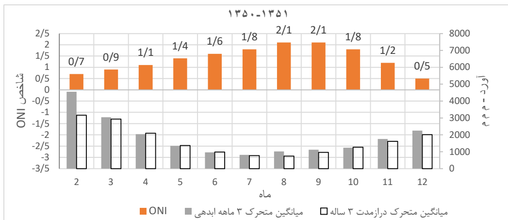
شکل (۶): میانگین متحرک ۳ ماهه و درازمدت ۳ ماهه‌ی آورد حوضه‌ی کارون و شاخص ONI در ال نینو سال ۱۳۵۰-۵۱
