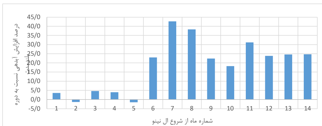
شکل (۱۳): میانگین درصد افزایش میانگین متحرک ۳ ماهه‌ی آبدی در دوره‌های ال نینو نسبت به میانگین بلندمدت
