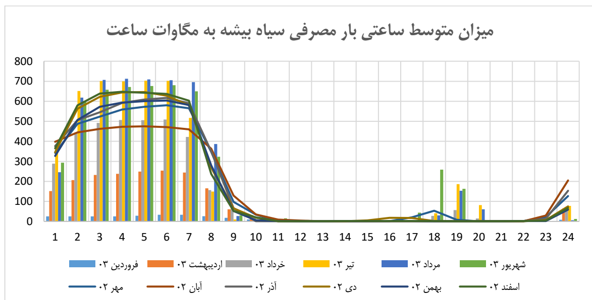
شکل (۳): میزان متوسط ساعتی بار مصرفی سیاه بیشه به مگاوات ساعت
