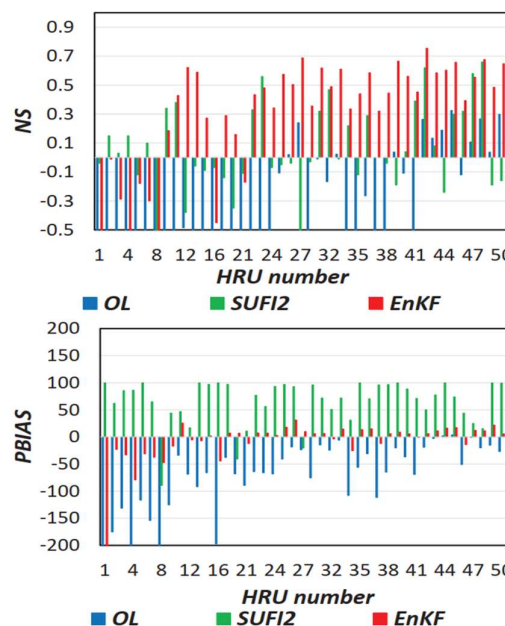
شکل ۴- مقدار معیارهای نکویی برازش در مقیاس هر HRU (a) معیار NS، (b) معیار PBIAS
