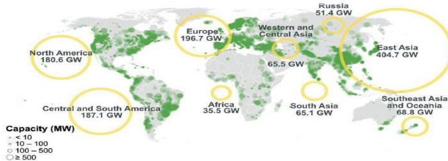
ظرفیت نیروگاه‌های تلمبه ذخیره‌ای عملیاتی در سال ۲۰۲۳
