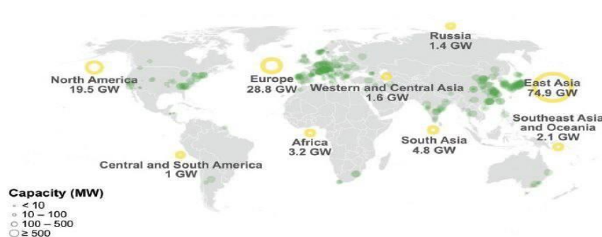
ظرفیت نیروگاه‌های تلمبه ذخیره‌ای عملیاتی در سال ۲۰۲۳
