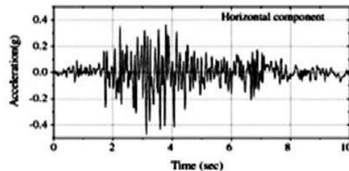
شکل (۴): مؤلفه‌ی افقی شتاب‌نگاشت زلزله کوبنا
