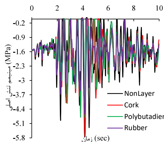
شکل (۹): منحنی پاسخ تاریخیچه زمانی تنش اصلی سوم در تراز شکستگی بدنه پایین‌دست سد (نقطه B)
