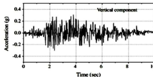
شکل (۵): مؤلفه‌ی قائم شتاب‌نگاشت زلزله کوبنا
