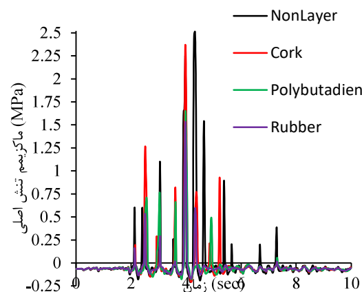
شکل (۸): منحنی پاسخ تاریخیچه زمانی تنش اصلی اول در تراز شکستگی بدنه پایین‌دست سد (نقطه B)
