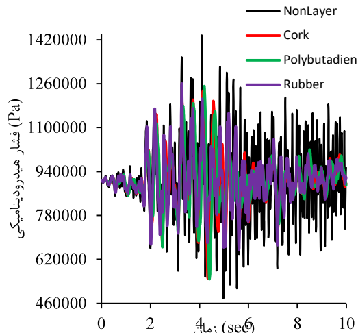
شکل (۱۲): منحنی پاسخ تاریخیچه زمانی فشار هیدرودینامیکی در نزدیکی پاشنه سد (نقطه C)
