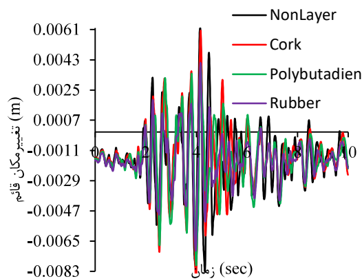
شکل (۱۱): منحنی پاسخ تاریخیچه زمانی تغییر مکان قائم تاج سد (نقطه A)
