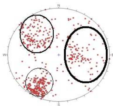
شکل (۵): کل قطب ناپیوستگی‌های برداشت‌شده به همراه تعداد ناپیوستگی در هر دسته و راستای خطوط برداشت با استفاده از نرم‌افزار Dips، دایره با ضخامت کم: لایه‌بندی، دایره با ضخامت متوسط: J_1 ، دایره با ضخامت زیاد: J_2
