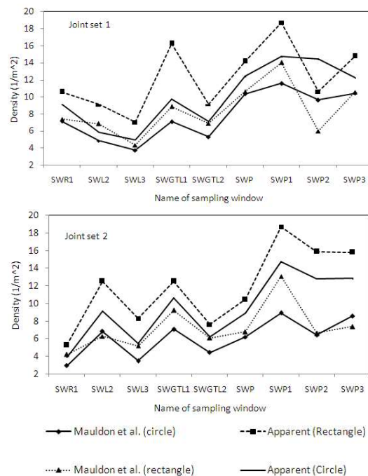
شکل (۱۱): چگالی سطحی واقعی و ظاهری دسته درزه‌های J 1 و J 2
