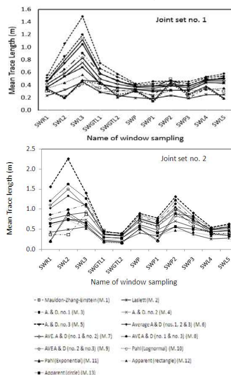
شکل (۷): نتایج میانگین طول اثر دسته درزه‌های J_1 و J_2 با استفاده از روابط مختلف
