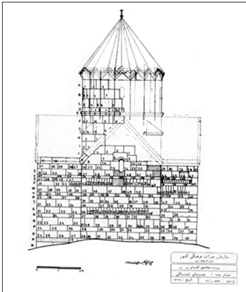
شکل (۱۲): طرح کدبندی سنگ‌ها برای پیاده‌سازی و بازچینی، با هدف احیاء بخش‌های تخریب‌شده. (طراح: مهندس وارژان آراکلیان)
