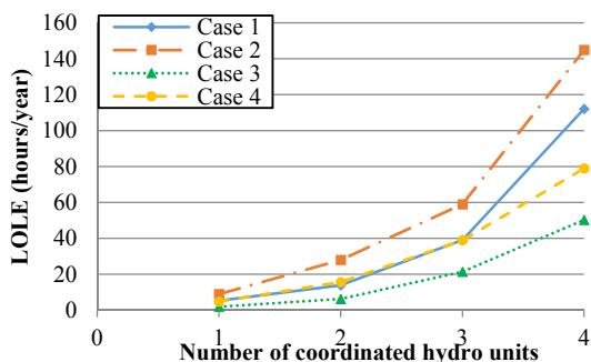
شکل (۳): میزان بار تأمین نشده انتظاری
