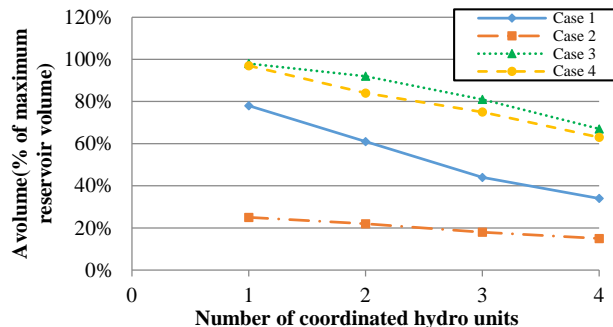
شکل (۶): حجم متوسط آب موجود در پشت سد
