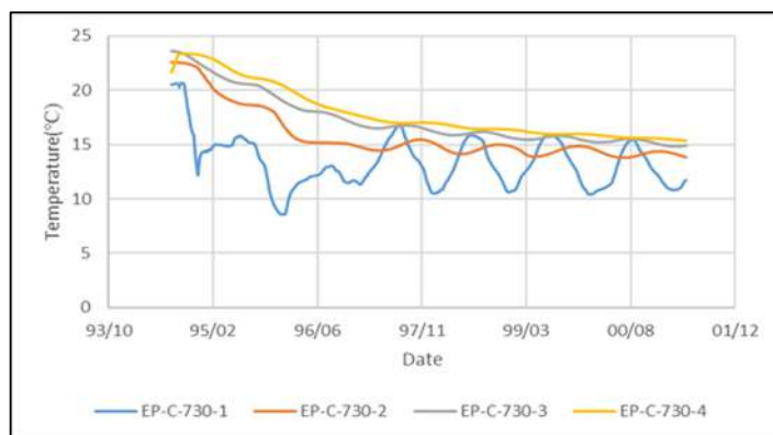
شکل (۹): تغییرات حرارتی ابزارها در تراز ۷۳۰ متر (کف هسته سد) در مقطع C
