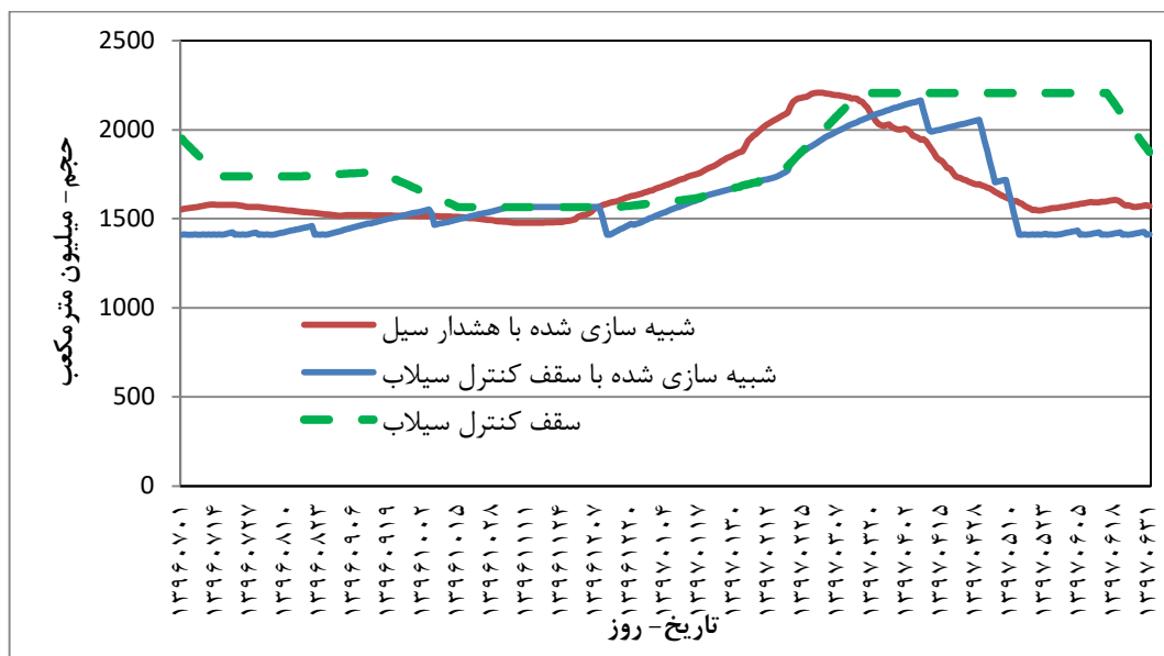
شکل (۴): مقایسه حجم مخزن رخ داده شده با سامانه‌ی هشدار سیل با حجم شبیه‌سازی شده بدون سامانه هشدار سیل در سال آبی خشک ۹۷-۱۳۹۶
