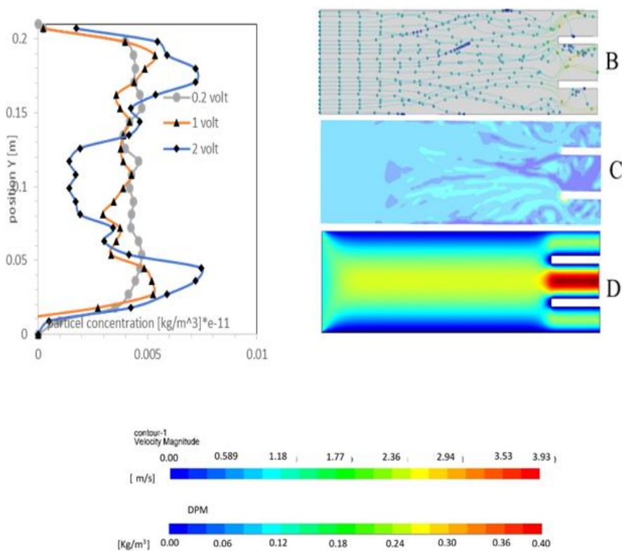
شکل (۸): A- میزان جدایش ذرات در خروجی در B=0.02 tesla، B- مسیر حرکت ذرات C- مقدار غلظت ذرات D- شمارگر سرعت
