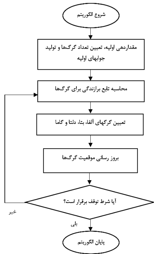
شکل (۲): فلوجارت کلی الگوریتم گرگ خاکستری
