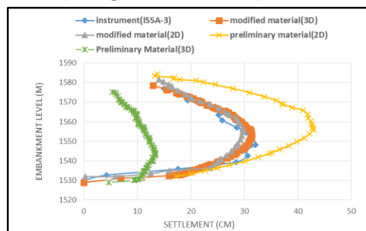
شکل (۸): مقایسه نشست پوسته پایین‌دست در فاصله ۲۸ متر از
