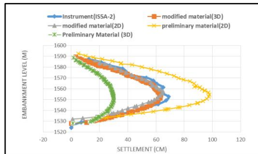
شکل (۷): مقایسه نشست هسته در فاصله ۶,۵ متر از محور سد
