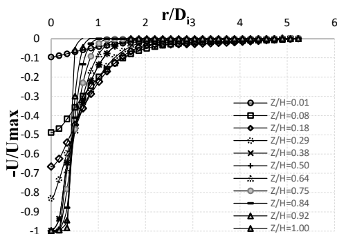
شکل (۱۲): نتایج مدل عددی برای پروفیل سرعت در ترازهای مختلف برای آزمایش شماره ۹ ( H=43 cm) (بر اساس شکل (۱) فاصله از کف حوضچه استغراق است)
