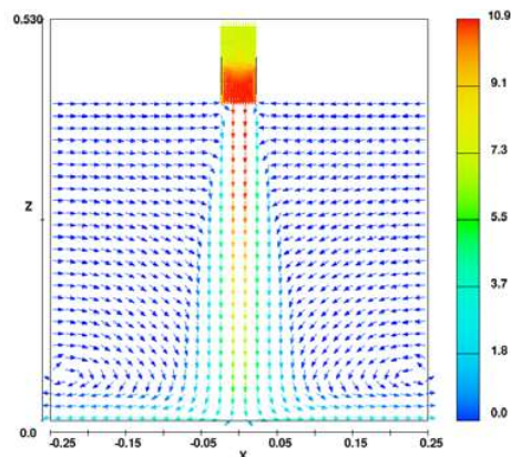
الف): میدان سرعت (بر حسب متر بر ثانیه)
