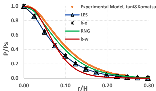
شکل (۶): مقایسه مدل‌های آشفتگی
