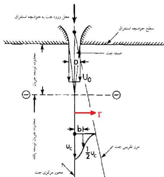
شکل (۳): مشخصات پروفیل سرعت در پخش جت در محدوده آزاد، برگرفته از راجاراتنام (۱۹۷۶)
