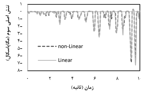
شکل (۱۴): مقایسه تاریخچه‌ی زمانی تنش اصلی فشاری برای دو حالت رفتار بتن بدنه سد
