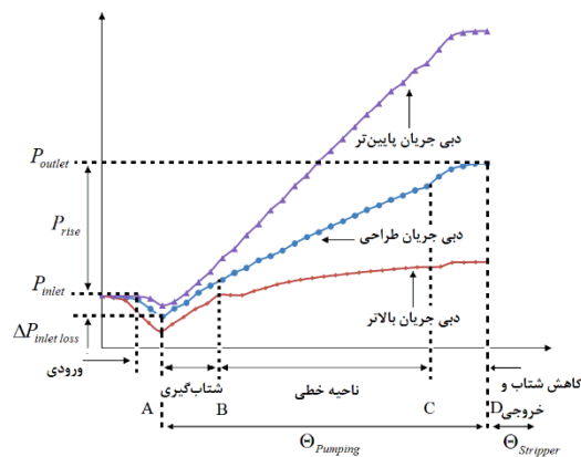
شکل (۱۴): تغییر فشار محیطی در پمپ رزنراتیو با پره‌های باکت‌مانند (تحلیل عددی)
