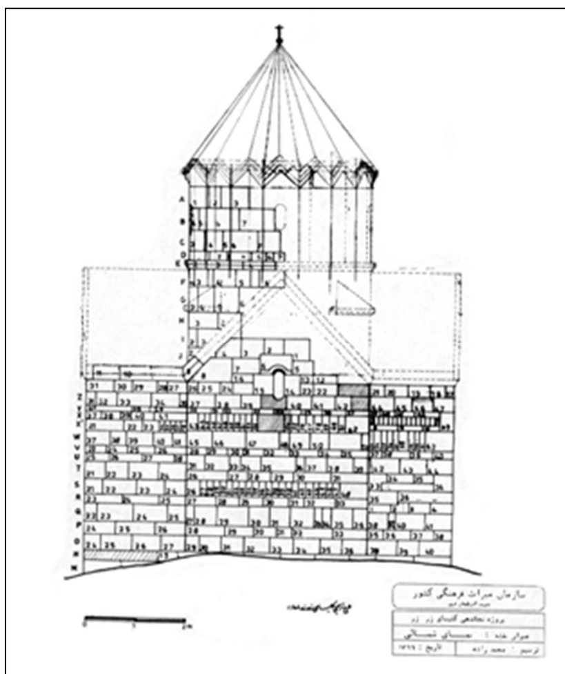
شکل (۱۲): طرح کدبندی سنگ‌ها برای پیاده‌سازی و بازچینی، با هدف احیاء بخش‌های تخریب‌شده. (طراح: مهندس وارژان آراکلیان)
