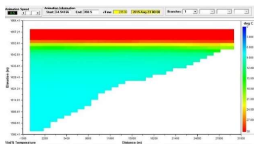
شکل ۴: نمای شماتیکی از لایه بندی حرارتی در مخزن کرخه در مدل CE-QUAL-W2
