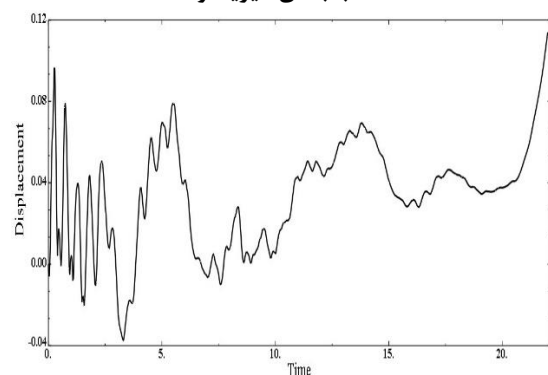
شکل (۹): نمودار جابجایی (متر) نقطه میانی روی سد (نقطه B) تحت شتاب‌های غیریکنواخت
