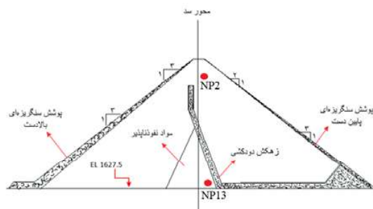
شکل (۹): نمایش مقطع عرضی سد درودزن در محور مرکزی سد به همراه موقعیت ۲ پیزومتر مورد مطالعه
